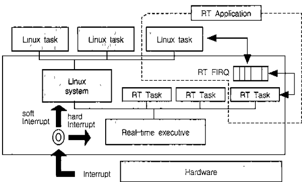
(그림 1) RT-Linux 구조
