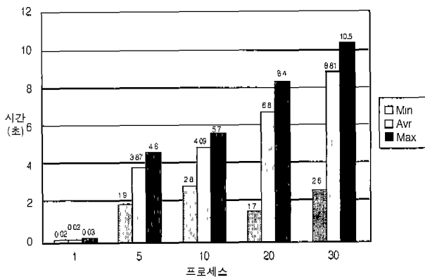
(그림 16) 테스트 4 결과표 : 왼쪽 막대부터 Min, Average, Max
