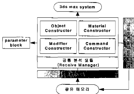
그림 11 수신측 모듈 구성도
