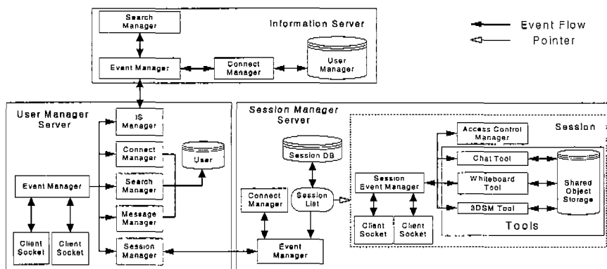
그림 1 협력 시스템 서버 구조
