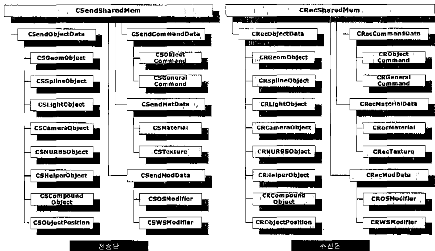
그림 7 공유 객체 송·수신을 위한 공유 메모리 관리 클래스
