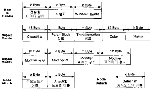
그림 6 플러그인과 공유 메모리간의 단계별 데이터 형식 정의
