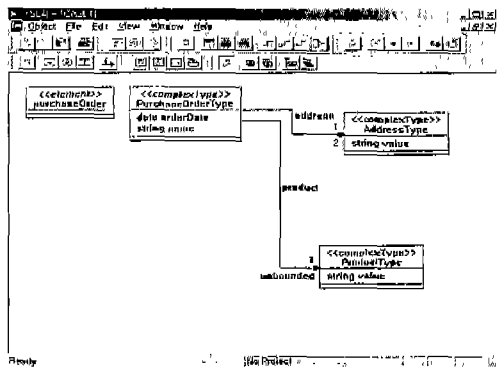
그림 10 PurchaserOrder 스키마
