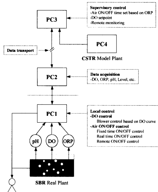
그림 3. 전체 플랜트제어 구성도.
