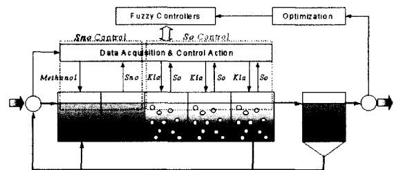
그림 1. CSTR 플랜트 제어를 위한 간략도.
