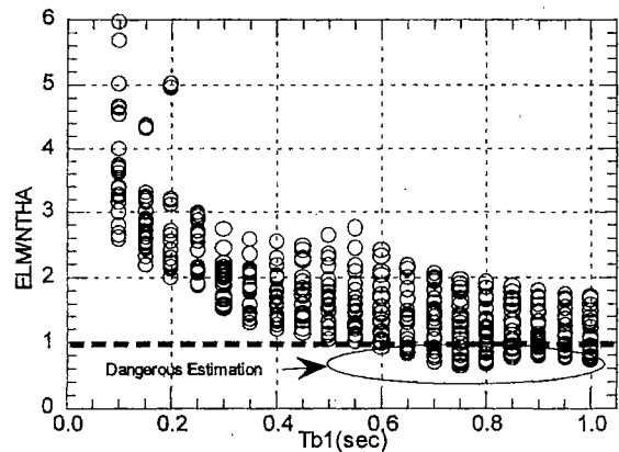
그림 3 일본건축학회의 식을 이용한 응답추정
