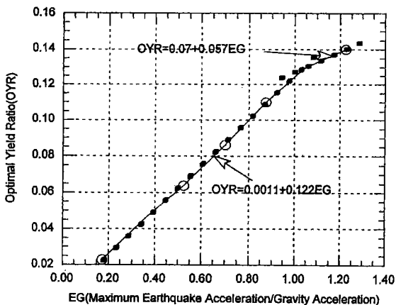
그림 6 지진력-최적항복비
