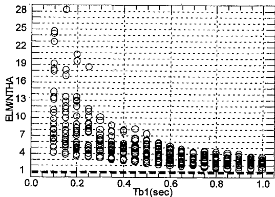
그림 1 일본도로교시방서의 식을 이용한 응답추정
