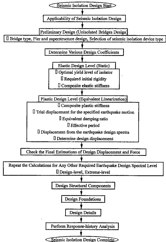
그림 7 TSID 설계 흐름도
