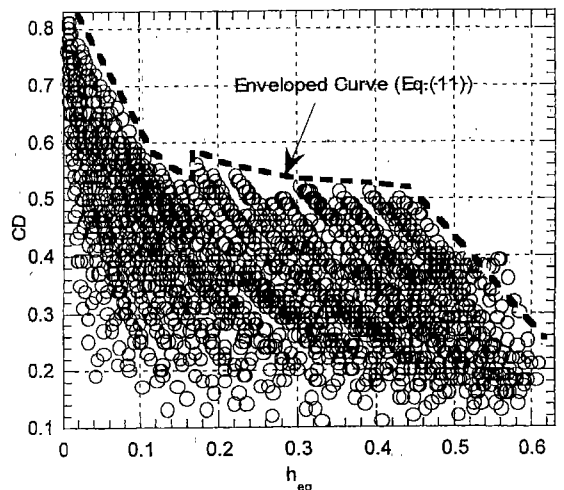
그림 4 등가감쇠비-비선형감쇠보정치
