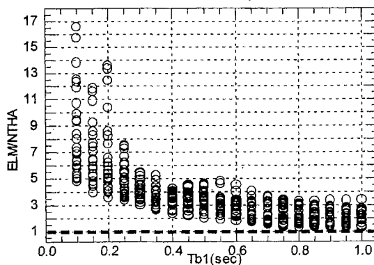
그림 2 K. Kawasima가 제안한 식을 이용한 응답추정
