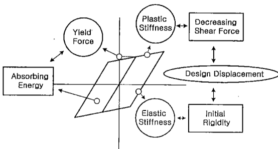
그림 5 바이리니어형 면진장치의 주요매개변수
