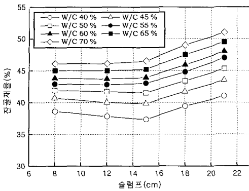
그림 2. 보통 콘크리트의 잔골재율(감자갈 25 mm)
