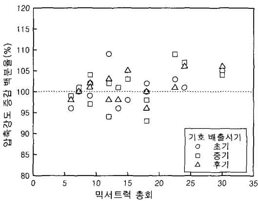
그림 8. 에지테이터 트럭 총 회전수와 압축 강도 증감 백분율
