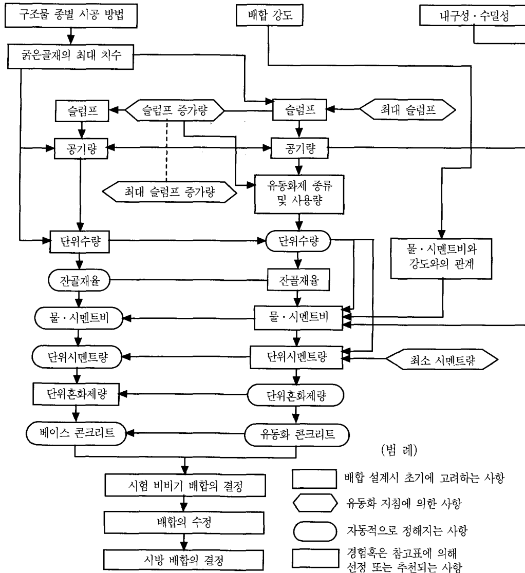
그림 1. 유동화 콘크리트의 배합 설계 흐름도
