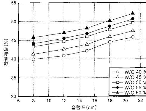
그림 5. 경량 콘크리트 2종의 잔골재율
