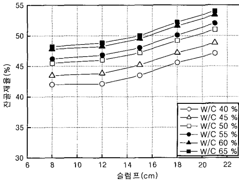
그림 4. 경량 콘크리트 1종의 잔골재율
