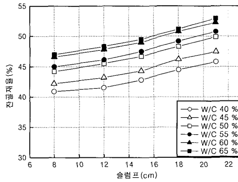
그림 3. 보통 콘크리트의 잔골재율(부순돌 20 mm)
