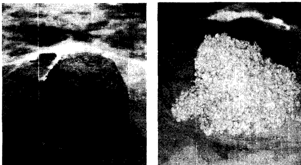
a) 유동화 전 b) 유동화 후 사진 1. 유동화 후 잔골재율 부족에 의한 재료 분리
