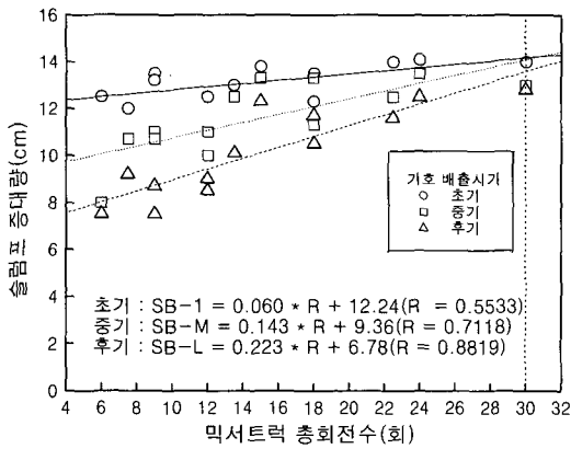
그림 6. 에지테이터 트럭 총 회전수와 슬럼프 증대량
