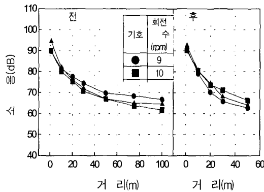
그림 9. 거리에 따른 소음의 변화
