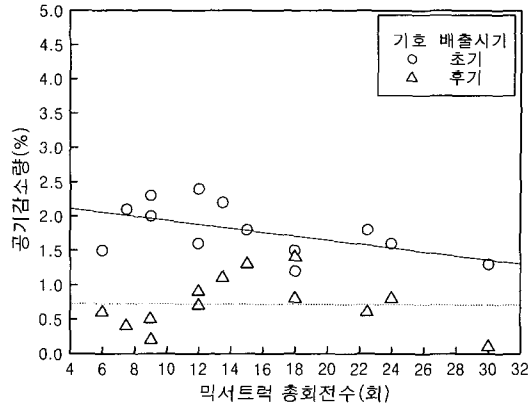
그림 7. 에지테이터 트럭 총 회전수와 공기 함소량
