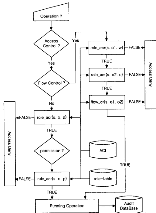
그림 1. 직무기반 접근제어 모델 구성도
