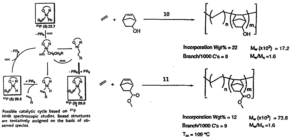
그림 11. Ni 촉매의 중합 메커니즘과 이를 이용한 관능기를 갖는 단량체와의 공중합.
