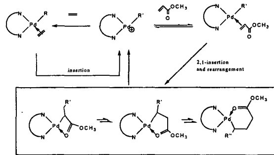
그림 10. Pd 촉매를 이용한 에틸렌과 MA의 공중합 catalytic cycle.
