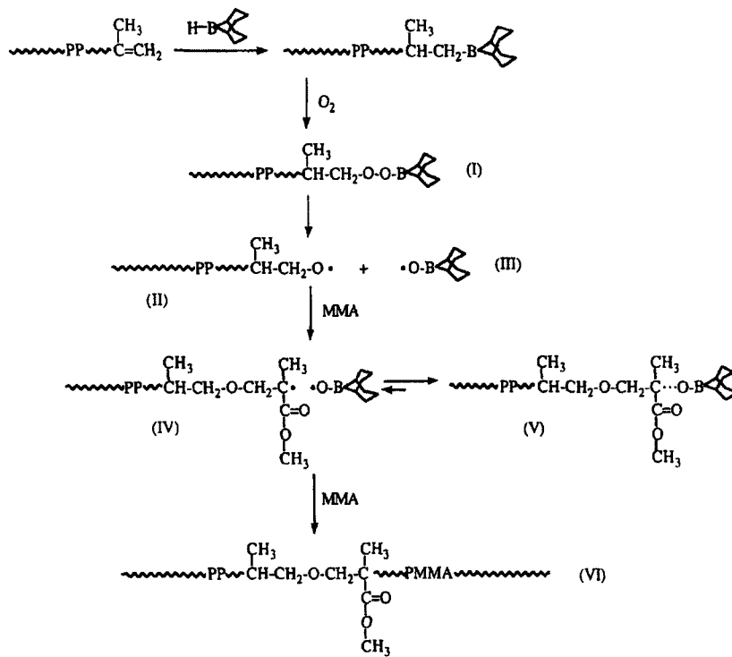
그림 2. Hydro-boration에 뒤이은 radical copolymerization을 이용한 PP-b-PMMA의 합성 메카니즘.
