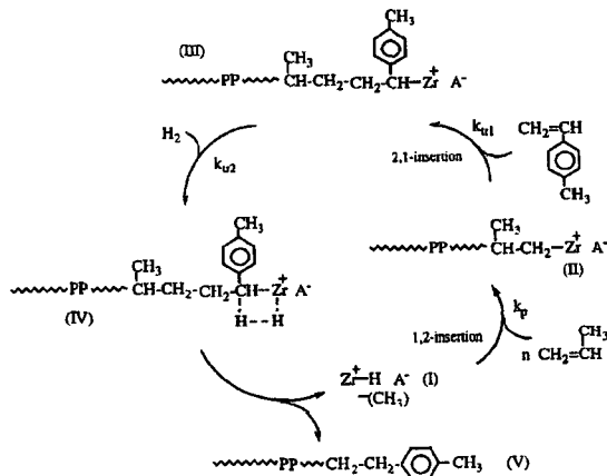
그림 9. 수소와 p -methyl styrene를 chain transfer agent로 사용하여 합성한 p -methyl phenyl functionalized PO의 catalytic cycle.
