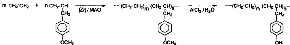
그림 5. Allylphenol과 ethylene의 공중합을 이용한 phenol group을 갖는 PE 합성.
