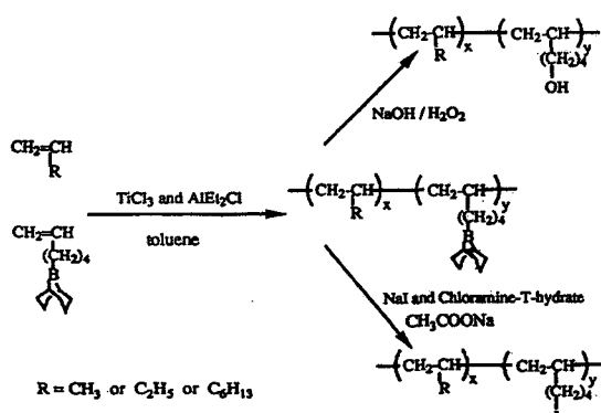
그림 6(a). 9-BBN protected 1,5-hexadiene을 이용한 관능기를 갖는 폴리올레핀 합성.
