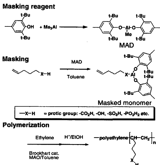
그림 6(b). MAD protected 단량체를 이용한 관능기를 갖는 폴리올레핀 합성.
