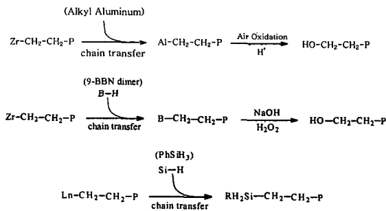
그림 8. End-functionalization에 사용된 chain transfer reactions.
