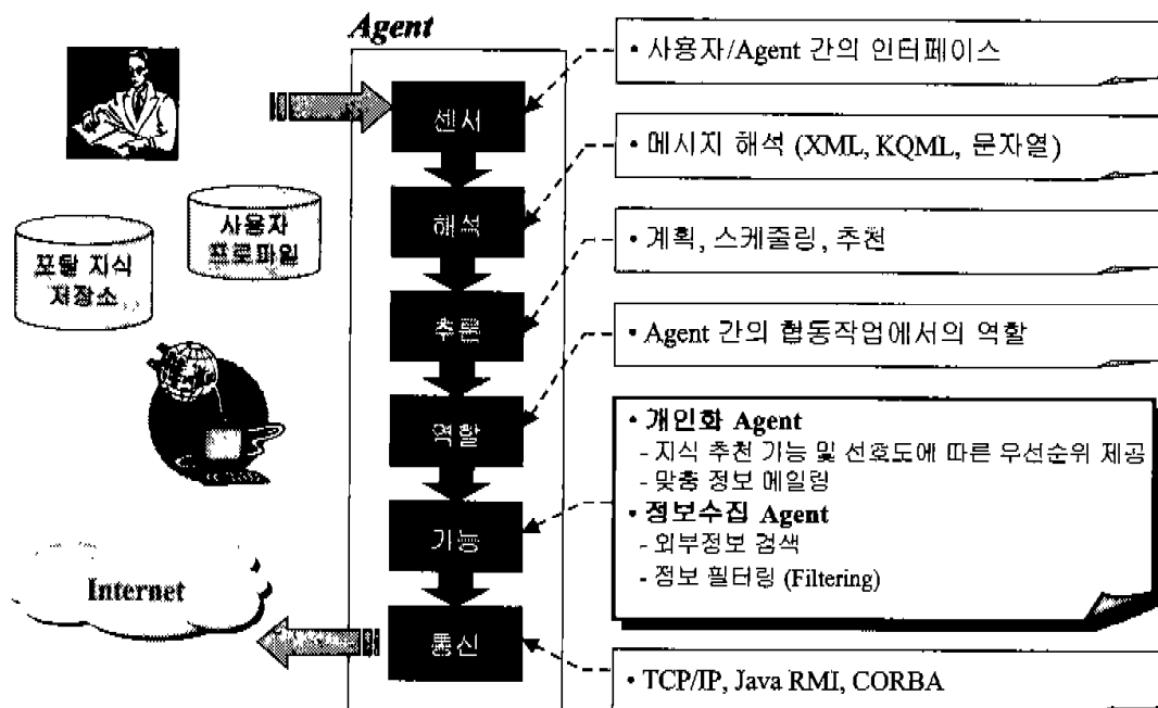
[그림 20. 개인화/정보수집 에이전트 개념도]
