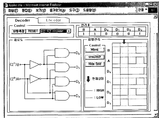
그림 4. 디코더/인코더의 동작원리 이해용 애플릿
