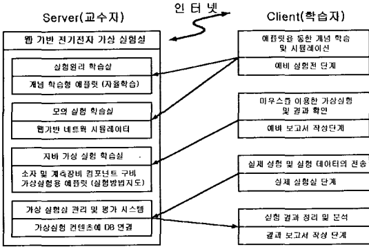
그림 1. 전기전자 가상실험실 학습모형의 개념도
