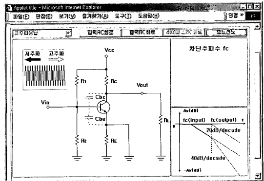
그림 3. 트랜지스터의 주파수특성 원리이해용 애플릿
