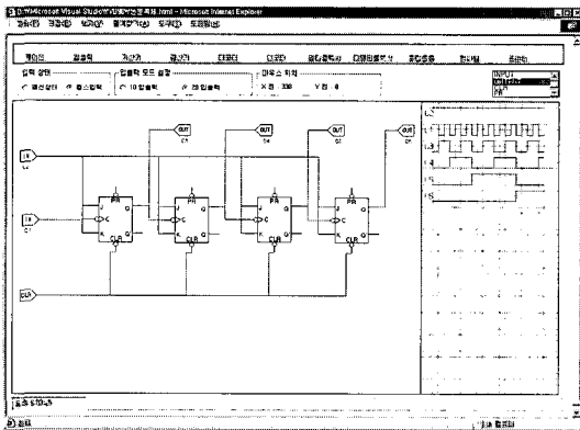
그림 5. 비동기식 업 카운터의 모의실험 실행화면
