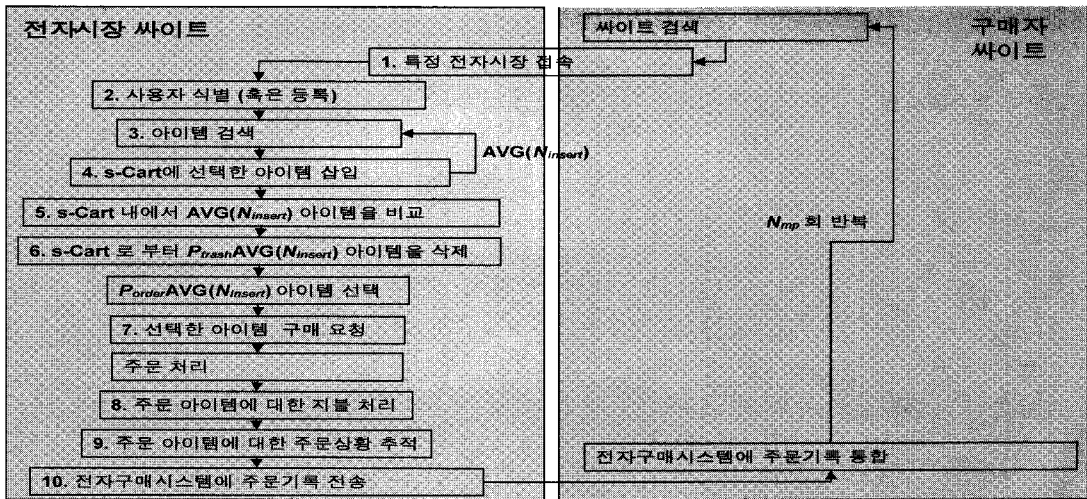
[그림 4] s-cart를 이용한 구매프로세스
