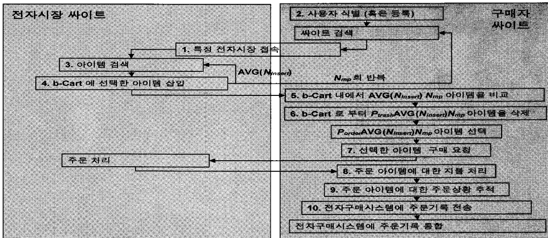
[그림 5] b-cart를 이용한 구매프로세스
