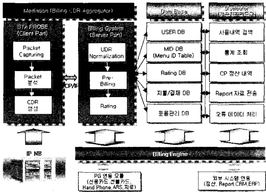
(그림 1) 과금 솔루션 소프트웨어 구조
