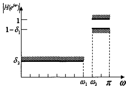
(b) HPF
