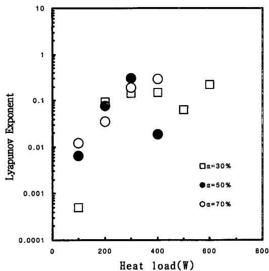
Fig. 12 Lyapunov exponent
