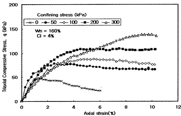
(a) ci=4%, Wi=160%
