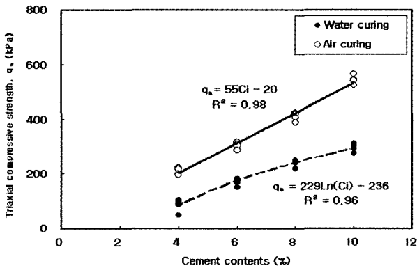
그림 7. 고화제 함유율에 따른 삼축압축강도 특성
