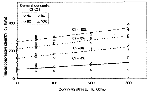
그림 8. 구속압 영향에 따른 압축강도특성
