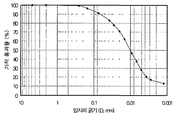
그림 1. 준설토의 입도분포 곡선
