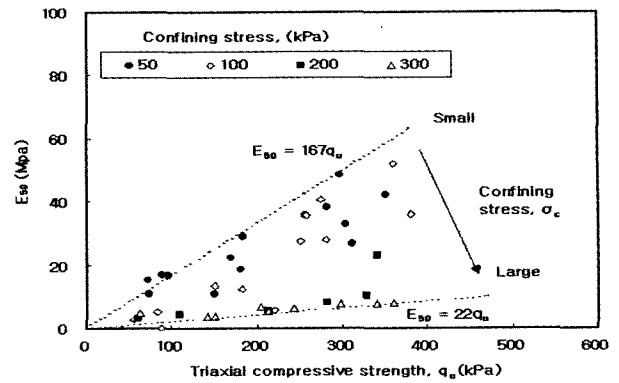
그림 10. 삼축압축상태의 압축강도와 할선 탄성계수의 관계
