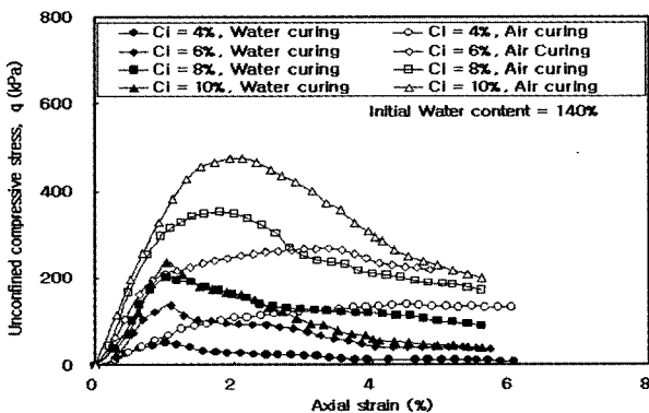
(a) 일축압축시험
