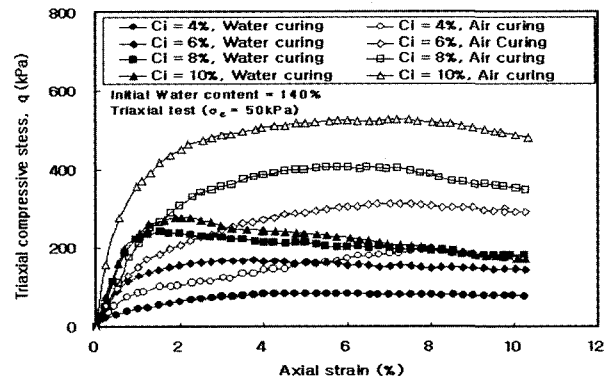
(b) 삼축압축시험( \sigma_c=50kPa )
