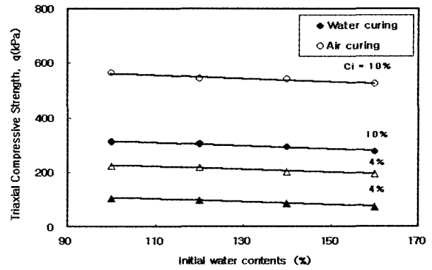
그림 6. 초기함수비에 따른 삼축압축강도 특성
