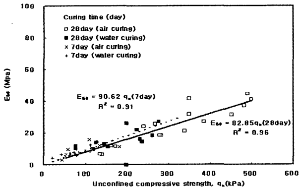
그림 9. 일축압축상태의 압축강도와 할선 탄성계수의 관계
