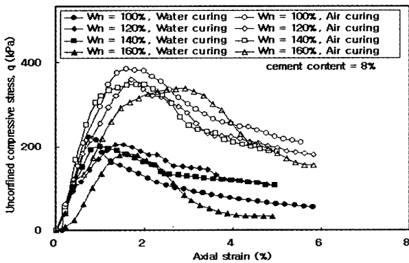
(a) 일축압축시험
