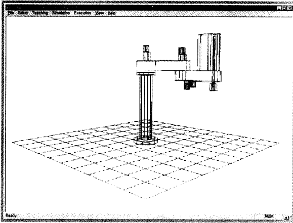
그림 10. 와이어 프레임 모델
