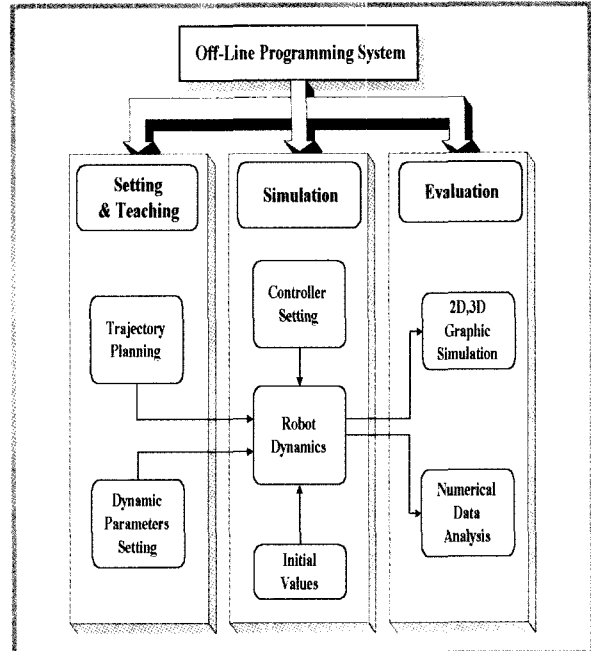
그림 2. 오프라인 프로그래밍 시스템의 구성
