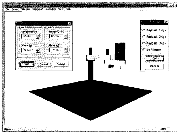
그림 5. Setup 메뉴의 Specification과 Payload 대화 상자
