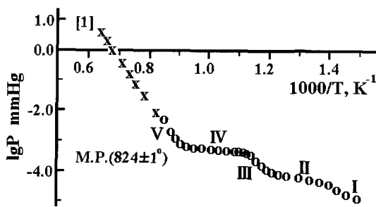
그림 8. \text{Bi}_2\text{O}_3 의 증기압과 온도와의 관계[6]. Fig. 8. The relation between the vapour pressure of \text{Bi}_2\text{O}_3 and temperature[6].
