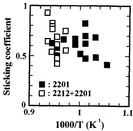
그림 5. 성막 온도에 대한 Sr 원소의 부착계수. Fig. 5. Sticking coefficient of Sr element vs. inverse temperature of the deposition.
