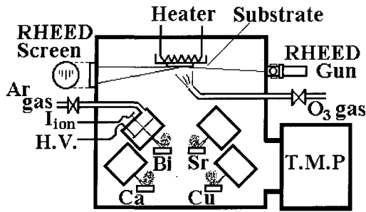
그림 1. IBS 시스템의 개략도. Fig. 1. Schematic diagram of the IBS system.
