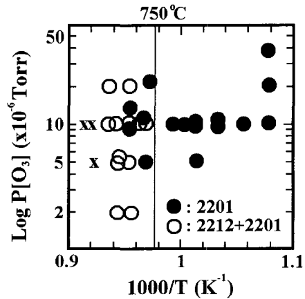
그림 2. 기관 온도와 오존 가스압에 대한 생성상도. Fig. 2. Phase diagram as a function of substrate temperature and ozone gas pressure.
