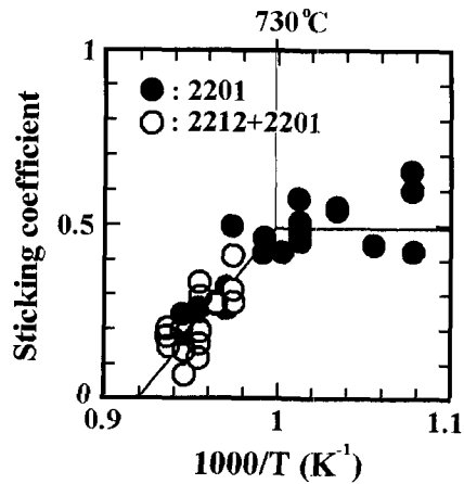
그림 7. 성막 온도에 대한 Bi 원소의 부착계수. Fig. 7. Sticking coefficient of Bi element vs. inverse temperature of the deposition.
