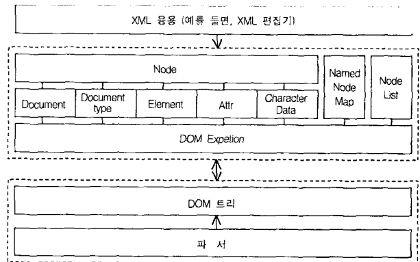
(그림 3) DOM 기반 XML 처리기의 구조
