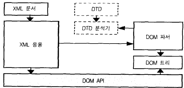
(그림 2) DOM 처리기의 동작 블록 다이어그램
