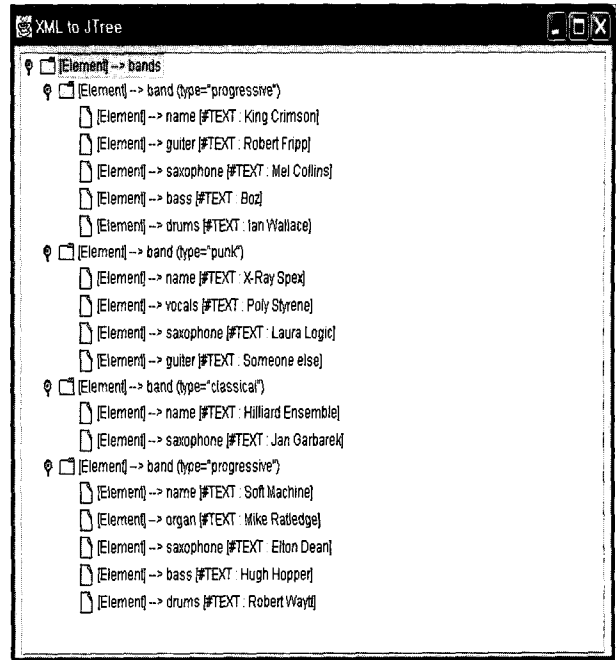
(그림 11) DOM 처리기(MM(9)) 응용 예
