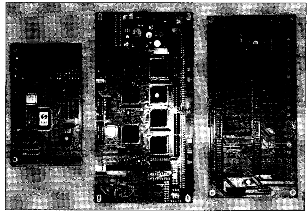
(그림 5) 개발된 시스템의 하드웨어
