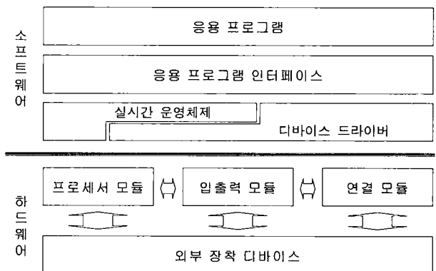
(그림 2) 범용 내장형 컴퓨터 시스템의 구조
