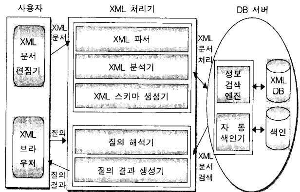
(그림 1) XML 문서 처리 과정
