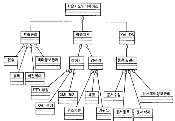
(그림 12) 학습지도 시스템의 개략적 클래스 다이어그램
