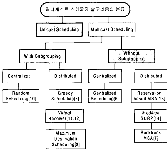
그림 2. 멀티캐스트 스케줄링 알고리즘의 분류 Fig. 2 Classification of Multicast Scheduling Algorithm
