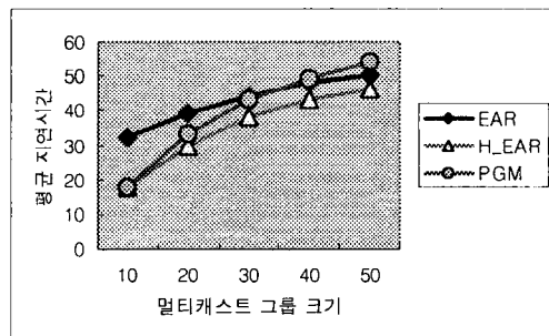
그림 11. 멀티캐스트 그룹 크기 vs. 평균지연시간 (L=3000) Fig. 11 Multicast Group vs. Average Delay Time (L=3000)
