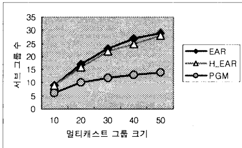
그림 10. 멀티캐스트 그룹 크기 vs. 서브그룹 수 (L=3000) Fig. 10 Multicast Group vs. Subgroup(L=3000)
