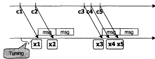
그림 4. EAR 알고리즘 Fig. 4 EAR Algorithm
