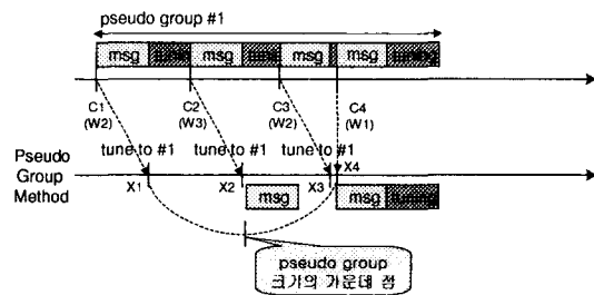
그림 7. Pseudo 그룹이 큰 경우 Fig. 7 Large Pseudo Group
