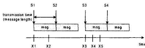
그림 3. EAR 알고리즘의 동작원리 Fig. 3 EAR Algorithm
