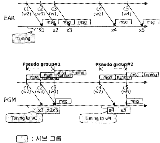
그림 6. EAR과 PGM 기법 비교 Fig. 6 EAR vs. PGM Algorithm
