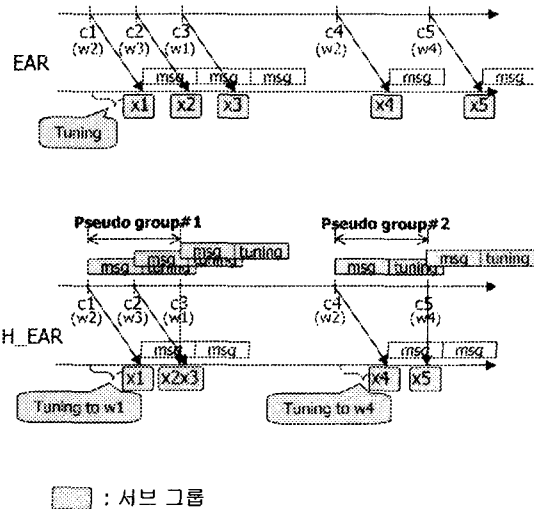
그림 5. EAR 알고리즘과 H-EAR 알고리즘 Fig. 5 EAR Algorithm vs. H-EAR Algorithm
