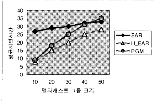
그림 9. 멀티캐스트 그룹 크기 vs. 평균지연시간 (L=1500) Fig. 9 Multicast Group vs. Average Delay Time (L=1500)
