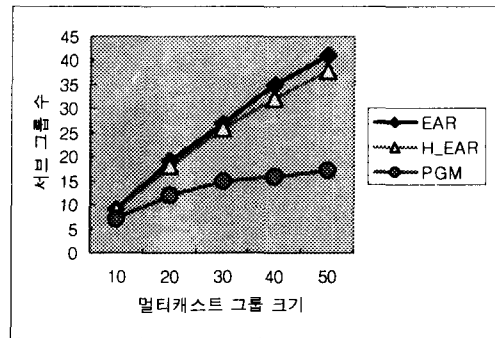
그림 8. 멀티캐스트 그룹 크기 vs. 서브그룹 수(L=1500) Fig. 8 Multicast Group vs. Subgroup(L=1500)
