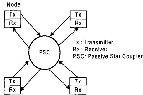
그림 1. WDM망의 구조 Fig. 1 Architecture of WDM Networks
