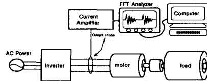
그림 1. 고장 진단 시스템 Fig. 1 Fault diagnosis system
