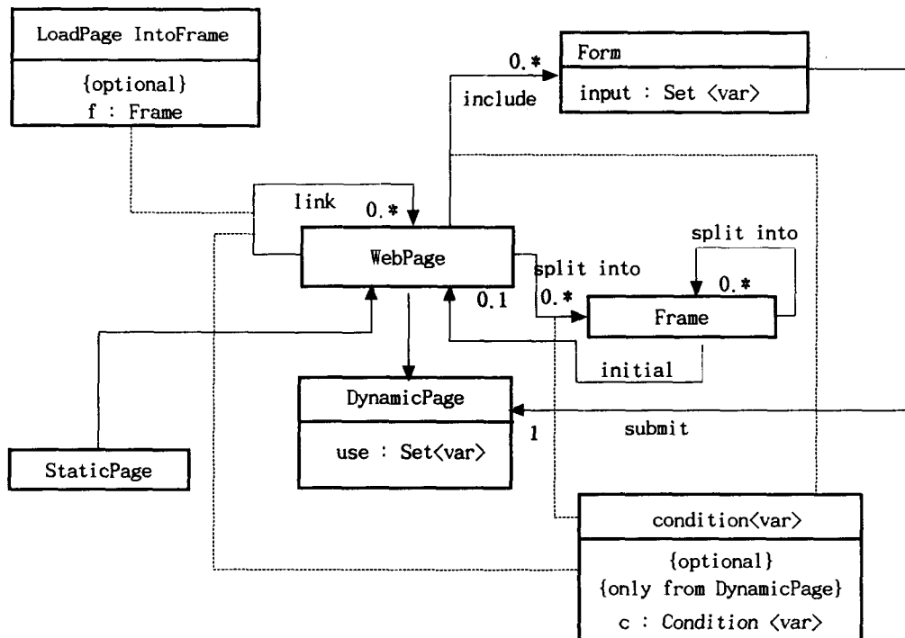
그림 1. 웹 어플리케이션 Meta model
