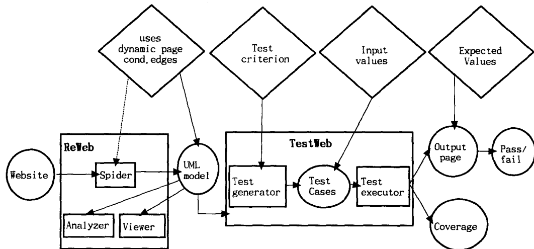
그림 4. ReWeb과 TestWeb의 역할
