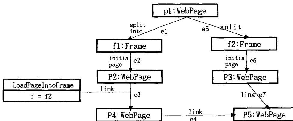
그림 2. 프레임들로 구성된 웹사이트 모델
