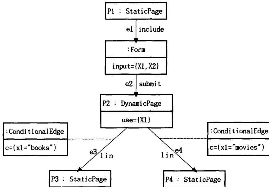
그림 3. 폼을 가지고 있는 웹페이지 모델
