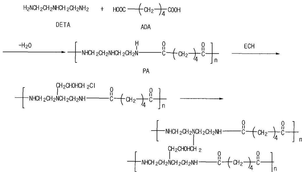
그림 2. Polyamide-amine 계열 탈수축진제 중합 반응.
