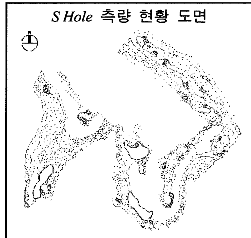
그림 2. 연구지역의 광파측량 현황도면
