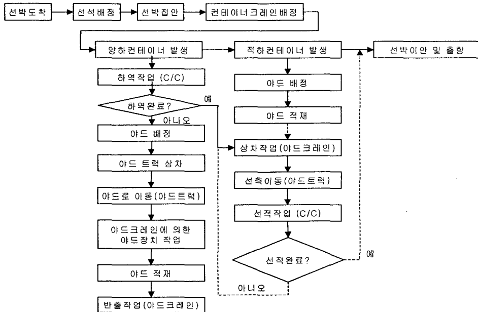
〈그림 3〉 컨테이너 터미널 작업 흐름도
