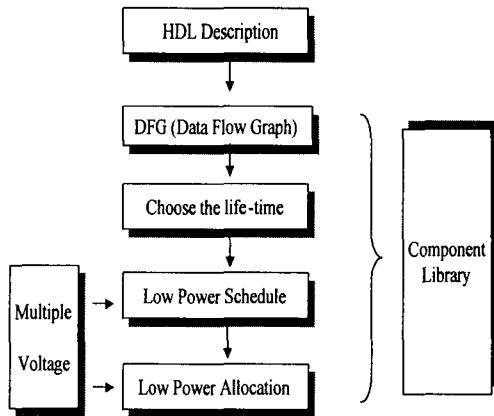
그림. 1 다중 공급 전압을 고려한 저 전력 스케줄링 및 할당 알고리즘 Fig. 1. Low power scheduling and allocation for multiple supply voltage
