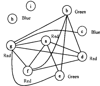
그림.12 최종적인 컬러링 그래프 Fig. 12. The final coloring graph
