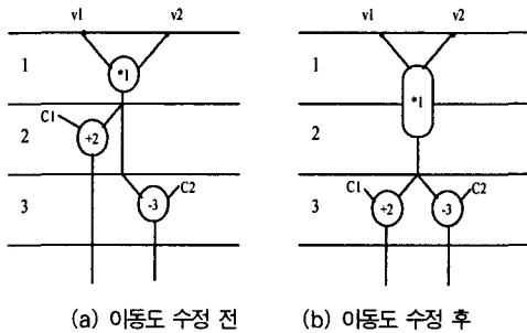
그림 9. 이동도 수정의 예 (a) Before the modification of mobility (b) After the modification of mobility Fig. 9. A example of modification the mobility
