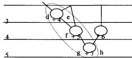
그림 8 기능연산자와 레지스터의 공유 Fig. 8 The sharing of functional unit and register
