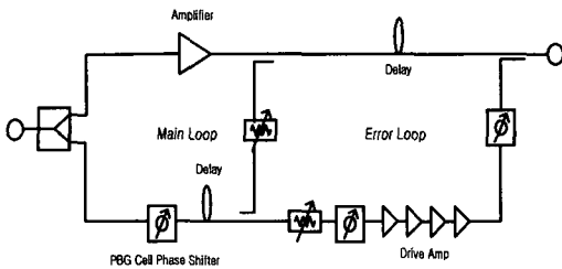
그림 4. Feedforward 선형증폭기에 적용된 천이격자 PBG
