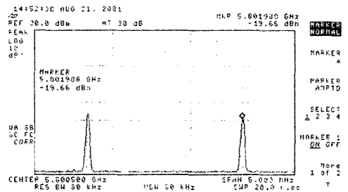
그림 6. PBG 천이격자를 이용한 주신호제거
