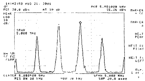
그림 5. 증폭기만의 IMD 특성
