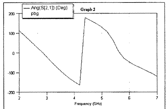
그림 3. PBG 격자 90° 천이된 위상특성
