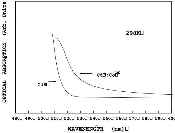
그림 4. 기초흡수단에서 CdS와 CdS:Co 2+ 단결정의 광흡수 스펙트럼(298K)
