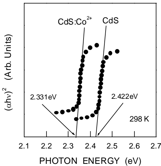
그림 5. CdS와 CdS:Co 2+ 단결정의 광학적 에너지 띠 간격(298K)
