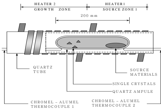
그림 1 화학수송법의 개략도 Fig. 1 Scheme of crystal growing CTR apparatus.
