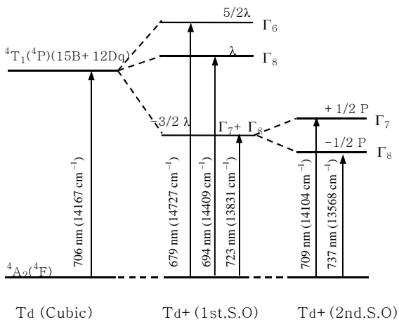
그림 7. CdS:Co 2+ 단결정내에서 Co 2+ 이온의 전자전이와 에너지 준위 분리(16K) Fig. 7. Energy-level splitting and electron transitions of Co 2+ ions in CdS:Co 2+ single crystals at 16K.
