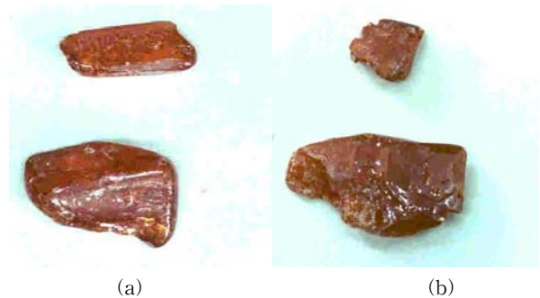
그림 3. 화학수송법으로 성장한 CdS와 CdS:Co 2+ 단결정의 사진 Fig. 3. Photographs of (a) CdS and (b) CdS:Co 2+ single crystals grown by the CTR method.
