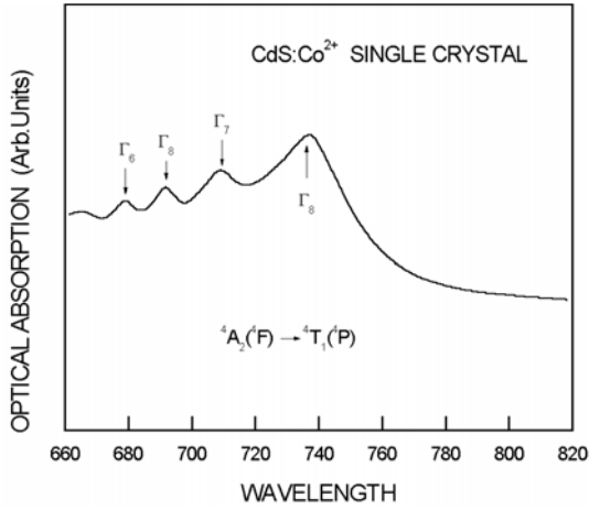
그림 6. CdS:Co 2+ 단결정내의 불순물 광흡수 스펙트럼(16K) Fig. 6. Impurity optical absorption spectrum of CdS:Co 2+ single crystals at 16K.
