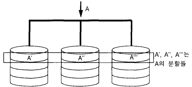
(그림 2) RAID 레벨 0
