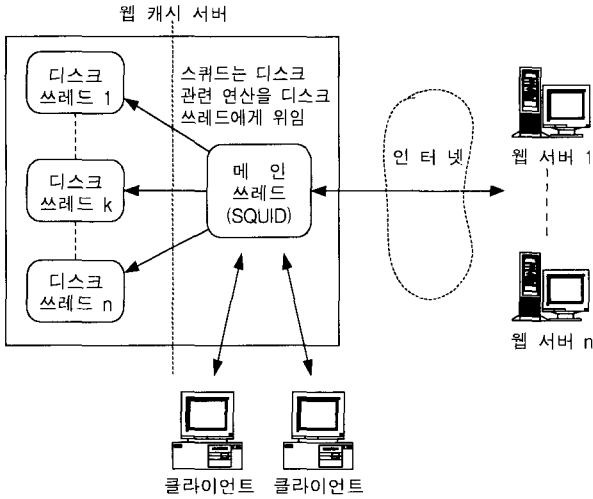
(그림 1) 디스크 쓰레드를 이용한 I/O 시간 중첩
