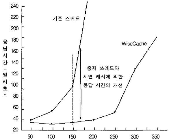
(그림 8) 기존 스쿼드와 WiseCache의 응답 시간 비교
