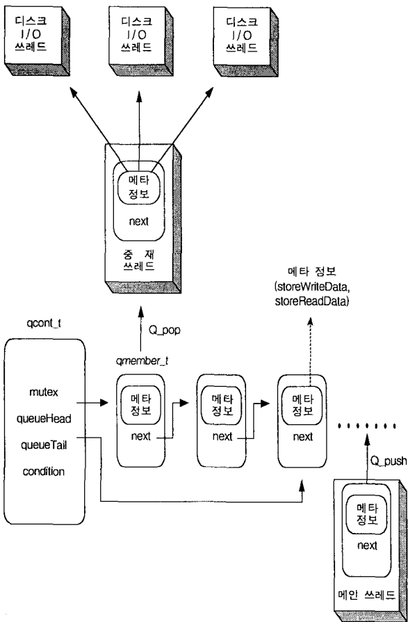
(그림 5) 중재 쓰레드를 이용한 WiseCache 동작 유형
