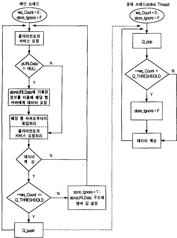
(그림 6) 지연 캐싱
