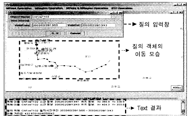
(그림 4) MPLength 연산자 수행 결과
