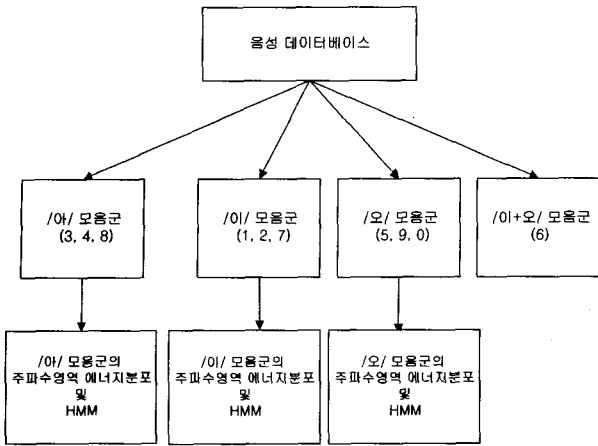
(그림 5) 모음 열을 추출하기 위한 기준모델 생성
