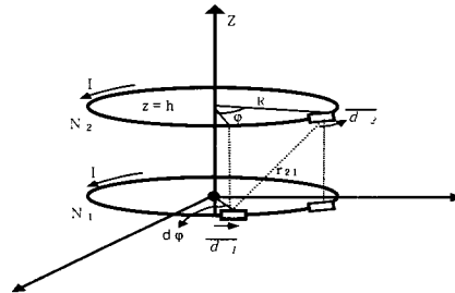
그림 3. 상호 인덕턴스 계산을 위한 코일 배치 Fig. 3. Coil arrangement for mutual inductance calculation.
