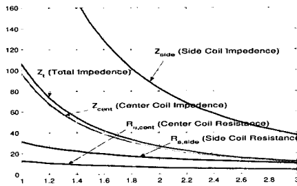
그림 8. 2軸 장치에서 \sqrt{2} mT 발생을 위한 인가 전류에 따른 임피던스(60 Hz 일 때) Fig. 8. Impedance by supplied current for \sqrt{2} mT generation in 2-axes device when it is 60 Hz.
