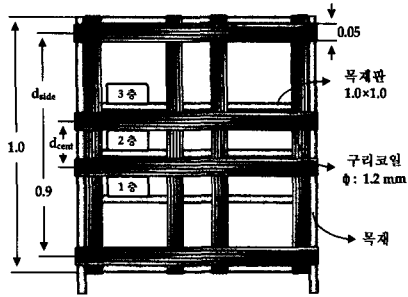
그림 4. 2축 자기장 발생장치의 설계도[m] Fig. 4. Schematic of 2-axes magnetic field generating apparatus[m].
