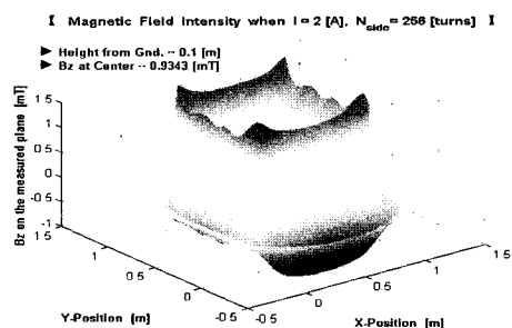
그림 12. z=0.1 m일 때의 B_z 분포 Fig. 12. Distribution of B_z on z=0.1 m plane.
