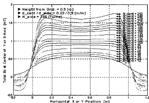
그림 11. 최적의 거리比와 권선比의 적합성 확인 Fig. 11. B_z at center point of y-or x-axis along horizontal x-or y-position with variable turns of N_{cent} .
