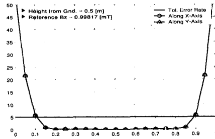
그림 20. z = 0.5 m 일 때의 편차율 Fig. 20. Error rate on z = 0.5 m plane.
