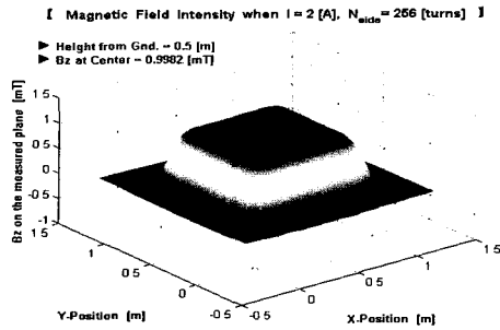
그림 16. z = 0.5 m 일 때의 B_z 분포 Fig. 16. Distribution of B_z on z = 0.5 m plane.
