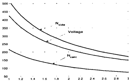
그림 7. 單軸 장치의 중앙점에서 1 mT 자기장 발생을 위한 전류, 권선數 및 인가전압(60 Hz 일때) Fig. 7. At a center point of a single axis device current, number of turns and impressed voltage for 1 mT magnetic field generation when it is 60 Hz.
