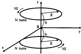
그림 1. 상하 두 개의 동일 복수 권선에 의해 자기장을 발생시키는 구조 Fig. 1. Structure of magnetic field source by the two same coils.
