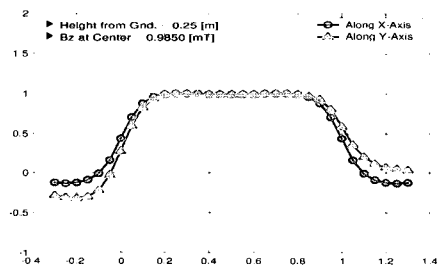
그림 15. 그림 14의 단면도 Fig. 15. Cross sectional view of Fig. 14.
