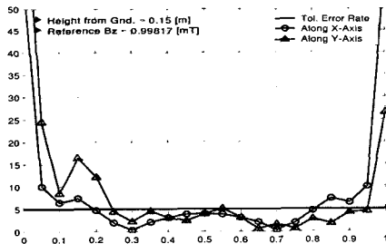
그림 18. z = 0.15 m 일 때의 편차율 Fig. 18. Error rate on z = 0.15 m plane.
