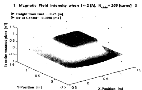
그림 14. z=0.25 m일 때의 B_z 분포 Fig. 14. Distribution of B_z on z=0.25 m plane.
