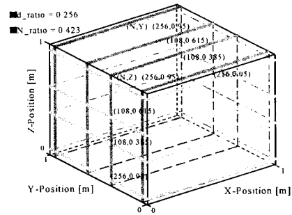
그림 10. 최적화를 통해 구해진 2軸 장치 구조도 Fig. 10. Structure of 2-axes device which was derived by optimization process.
