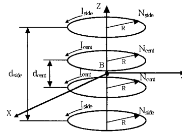
그림 2. 권선수가 다른 4중 코일에 의해 자기장을 발생시키는 구조 Fig. 2. Structure of magnetic field source by the fourfold coil whose number of turns differ.
