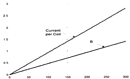
그림 9. 單軸 장치에서 N_{side} = 256 , N_{cent} = 108 일 때 인가전압에 따른 자속밀도 및 전류의 변화 Fig. 9. Change of magnetic flux density and current by impressed voltage when N_{side} = 256 and N_{cent} = 108 in a single axis device.
