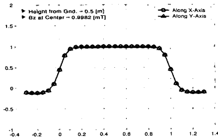
그림 17. 그림 16의 단면도 Fig. 17. Cross sectional view of Fig. 16.
