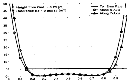
그림 19. z = 0.25 m 일 때의 편차율 Fig. 19. Error rate on z = 0.25 m plane.
