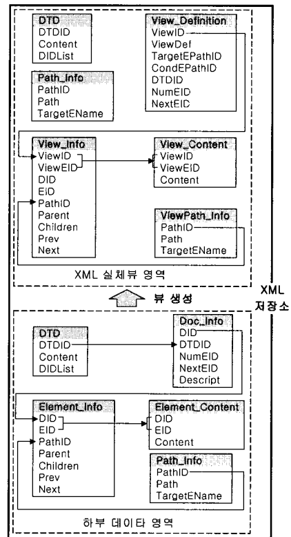
(그림 4) XML 저장소의 테이블 스키마
