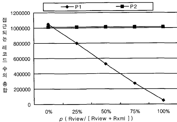
(그림 20) 비율 p 의 변화에 따른 레코드 접근 회수
