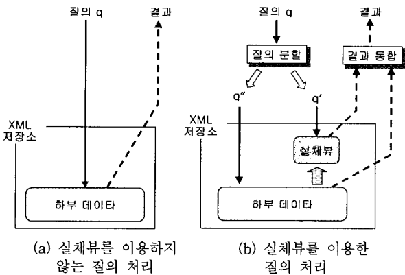
(그림 1) XML 저장소를 대상으로 한 질의 처리
