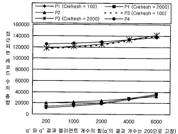
(그림 18) 결과 엘리먼트 개수의 변화에 따른 레코드 접근 회수
