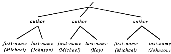
(a) 트리 형태로 표현된 XML 실체뷰
