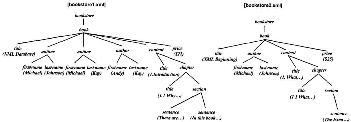
(그림 2) 하부 데이터에 저장된 XML 문서의 예
