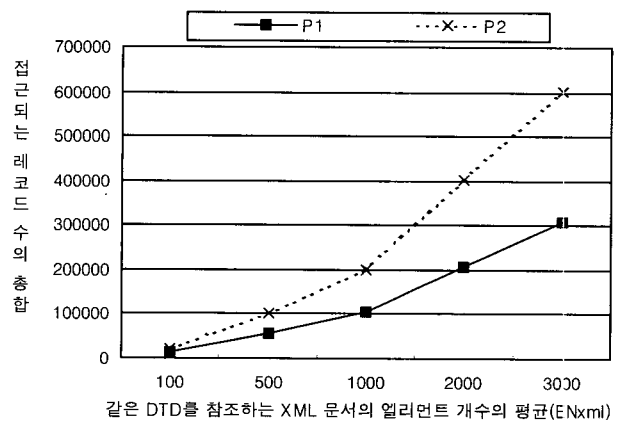
(그림 19) XML 문서의 엘리먼트 개수의 변화에 따른 레코드 접근 회수
