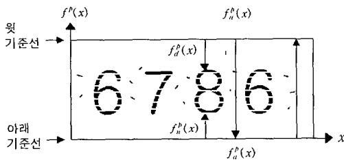
(그림 15) 예지 값 형성 기준치
