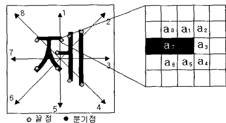
(그림 17) 개선된 Field Effect 기법
