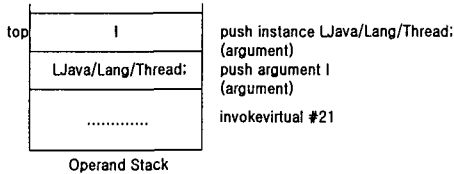
그림 10. 메소드 호출 명령을 위한 Operand 스택과 명령어 순서
