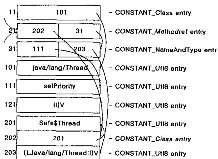
(a) Thread.setPriority(I)V에 의한 수정
