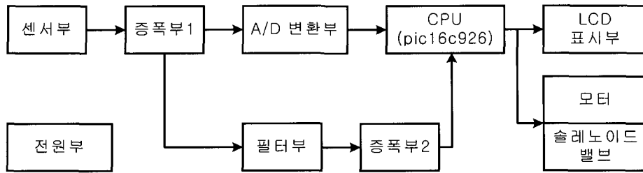
그림 1. 상완혈압/두부혈압 측정시스템의 구성도 Fig. 1. Block diagram of BP/HBP measurement system
