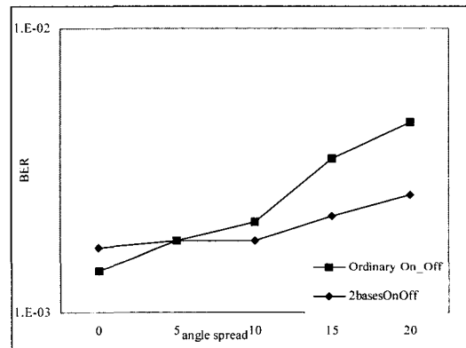
그림 5. 파워 비율이 같음(PG=256)때의 BER 성능 Fig.5. BER performance when Power ratio is equal(PG=256)
