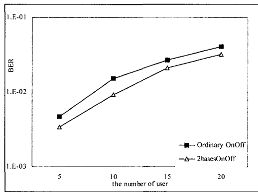
그림 8. 각도퍼짐이 20^0 (PG=256)일 때의 BER 성능 Fig.8. BER performance when angular spread is 20(PG=256)
