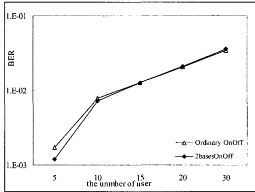
그림 7. 각도퍼짐이 10^0 (PG=256)일 때의 BER 성능 Fig.7. BER performance when angular spread is 10(PG=256)
