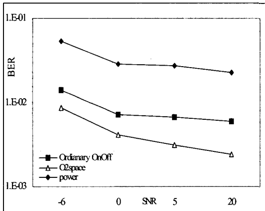
그림 12. SNR 따른 Power Method과의 BER 비교 성능(PG=64) Fig.12. BER performance with Power Method(PG=64)
