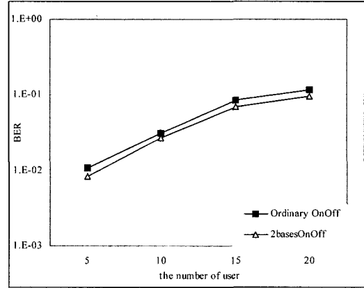
그림 9. 각도퍼짐이 10^0 (PG=16)일 때의 BER 성능 Fig.9. BER performance when angular spread is 10(PG=16)
