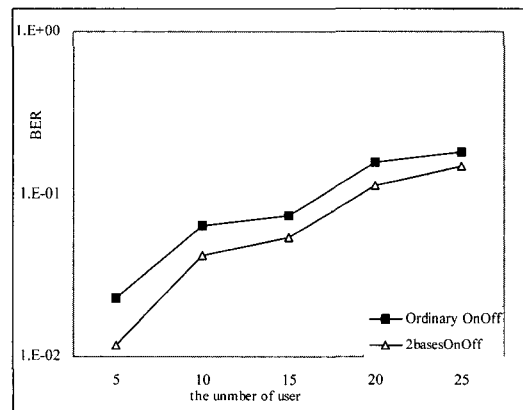
그림 10. 각도퍼짐이 20^0 (PG=16)일 때의 BER 성능 Fig.10. BER performance when angular spread is 20(PG=16)
