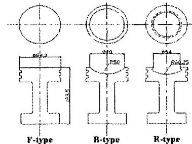
(b) Piston type
