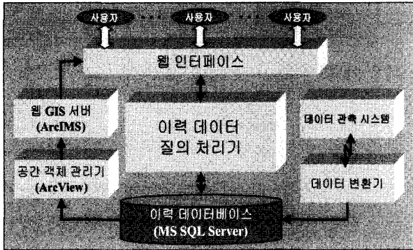
(그림 1) 대체에너지원 이력 데이터 관리 시스템 구조
