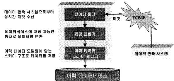
(그림 2) 데이터 변환기
