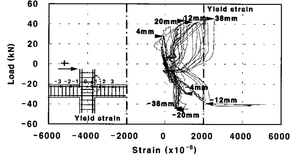
(d) Location 1 (model 4)
