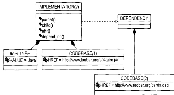
(그림 11) IMPLEMENTATION(2)의 클래스 다이어그램
