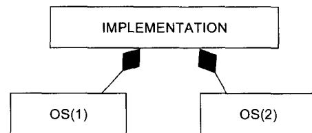
(그림 2) [규칙 1]의 클래스 다이어그램
