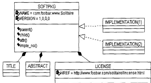
(그림 10) SOFTPKG의 클래스 다이어그램
