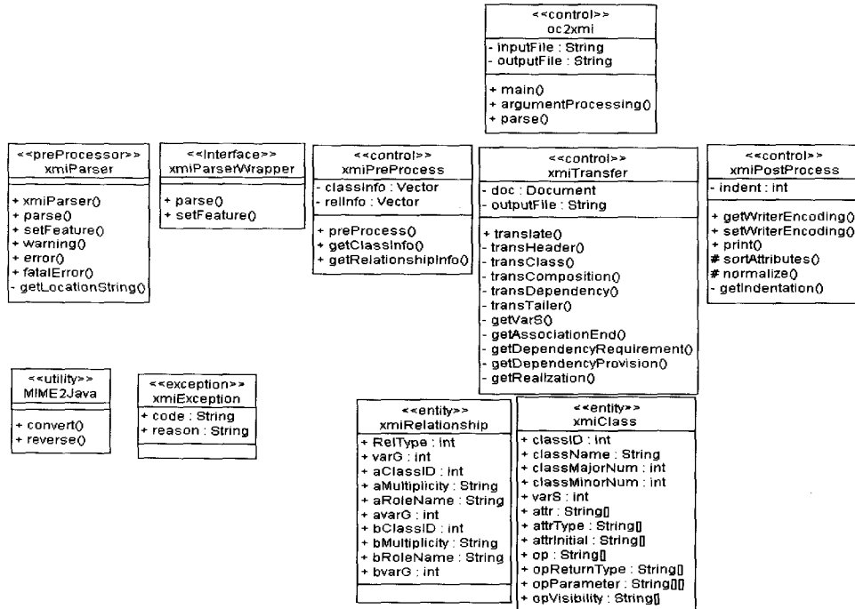
(그림 8) (그림 7)의 주요 클래스들
