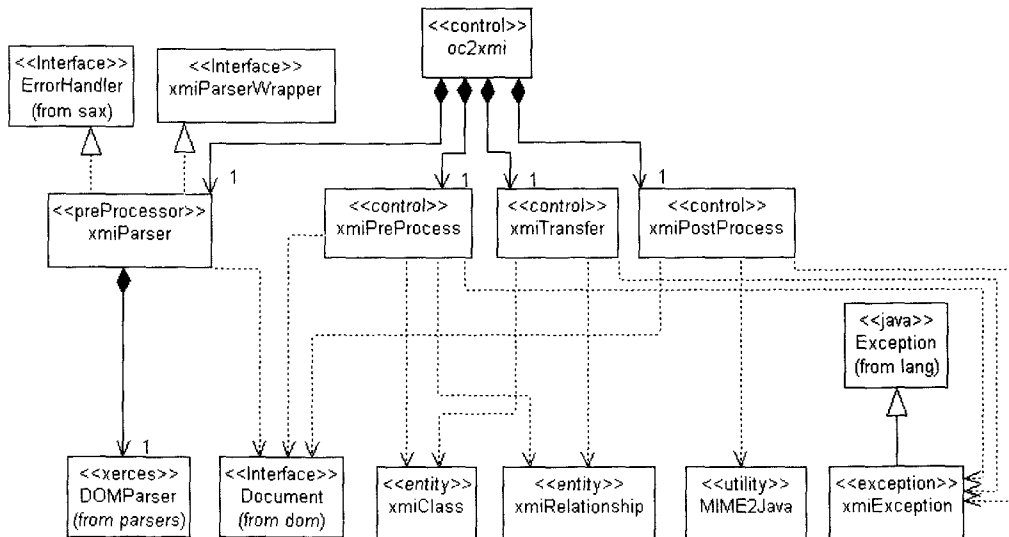
(그림 7) XMI 문서 생성을 위한 클래스 다이어그램
