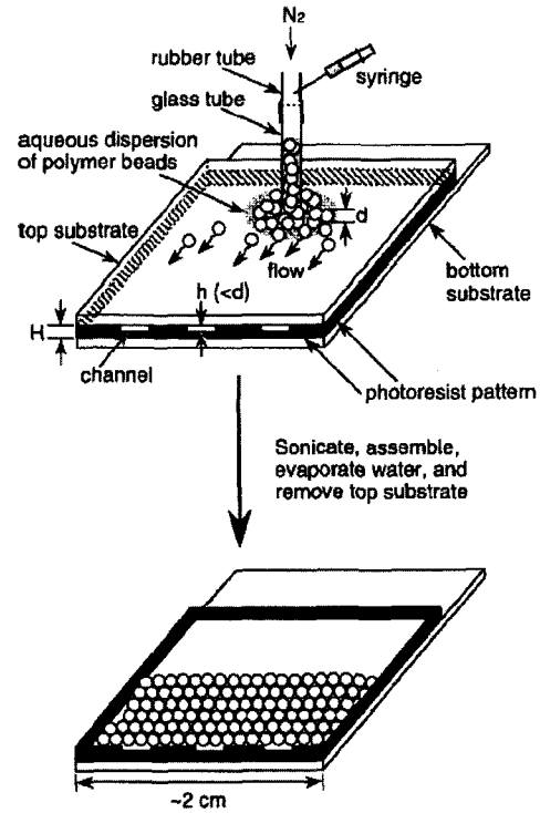
그림 9. 폴리스티렌의 분산액을 실린지를 이용하여, 고무 튜브를 통해 셀 안으로 주입한다. 고분자 입자들의 퇴적 속도는 질소의 압력이 증가할수록 증가한다. 69
