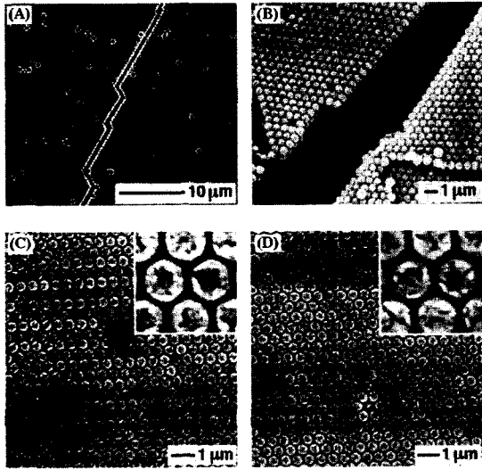
그림 10. 0.48\ \mu\text{m} 크기의 폴리스티렌 입자를 두께가 12\ \mu\text{m} 인 셀 안에 배열한 3차원 결정의 전자현미경 사진; (A) 위에서 본 결정 모양; (B) 선 결함에 대한 확대 사진; (C, D) 결정의 최상 및 최하층에 대한 사진. 69
