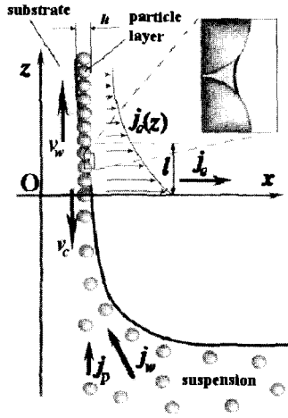
그림 5. 현탁액으로부터 끌어올려지는 기질 위에서 성장하는 단층의 입자 배열의 근처에서의 입자와 물의 흐름. 23
