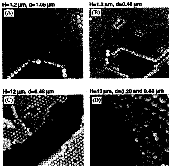
그림 11. 입자 크기( d ) 및 셀 두께( H )에 따른 배열 사진; (A) 단층; (B) 2중층; (C) 약 25개의 층으로 구성된 다층; (D) 두 가지의 크기를 가진 입자를 이용하여 배열된 층의 경계면. 69
