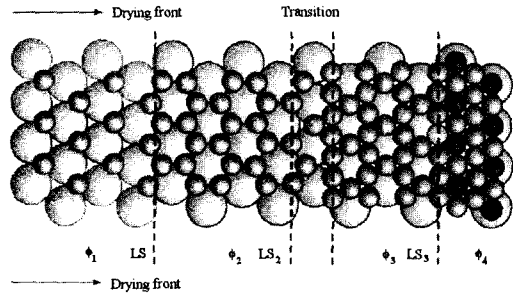
그림 13. 2원적 콜로이드의 배열( \gamma=0.5 )에서 크기 작은 입자의 배열 특성에 관한 모식도; 작은 입자들이 육모체의 2차원적 배열을 하며, 부피 분율( \Phi )에 대한 함수로 배열 특성 LS에서 LS 2 , LS 3 로 달라지게 된다. 81
