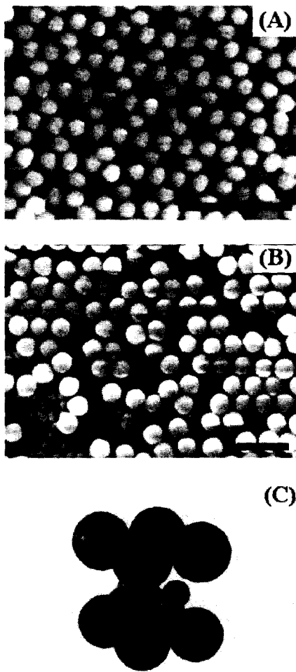
그림 12. 양큰비가 LS 3 인 2원적 3차원 콜로이드 결정; (A) LS 3 형의 2차원 배열 형태를 가지는 결정에서 입자의 크기가 작은 부분이 위로 배열된 층을 확대한 사진 (bar = 1 \mu m); (B) (A)의 층을 텀플레이트로 하여, 큰 입자를 부분적으로 배열된 층의 사진; (C) LS 3 형 결정의 모식도. 81
