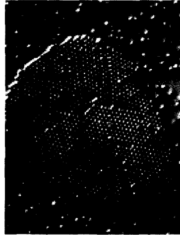
그림 6. 반대 전하를 띤 베시클과 콜로이드 입자들의 상호작용에 의해서 형성된 2차원 콜로이드 결정. 47
