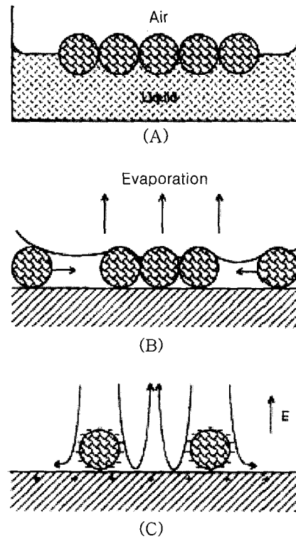
그림 1. 단분산 콜로이드의 2차원적 육모꼴 (hexagonal) 배열에 관한 개략도; (A) 긴 범위의 인력작용에 의한 공기-액체 계면에서의 배열; (B) 고체 기질 위에 퍼진 얇은 액체의 삼투압 인력에 의한 배열; (C) 고체 전극의 표면의 전기영동 퇴적에 의한 배열. 69
