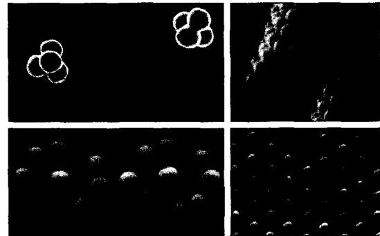
그림 8. 다른 제한 조건에서의 입자 퇴적; (왼쪽 위) 사면체의 사면체 클러스터들은 에멀전 방울에 닿아있는 건조되는 입자에 의해서 형; (오른쪽 위) 두 벽사이에 입자들이 쌓임으로써 야기되는 프리즘 상; (왼쪽 아래) 고분자 층의 구멍은 입자들이 모이는 용기로서 작용; (오른쪽 아래) 큰 입자들 위에 작은 입자들의 규칙적인 배열은 층겹침 방식으로 건조되면서 생성. 90
