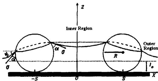
그림 4. 수평의 고체 기질 위의 액체 층에 부분적으로 잠겨있는 두 입자. 액체-기체 계면에서의 메니스커스의 변형은 입자 간의 인력을 증가시킨다. 22
