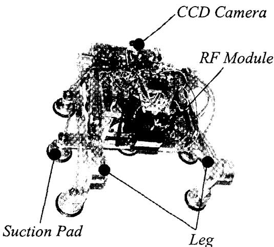
Fig. 1 MRWALLSPECT-II
