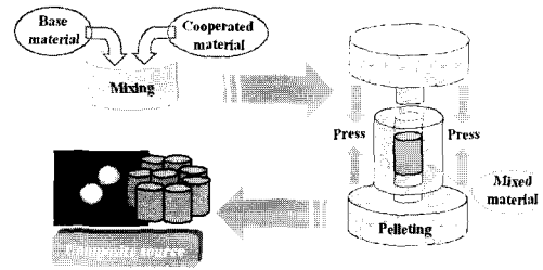
그림 1. 토대가 되는 무기물과 다른 무기물을 소량 첨가한 무기물 제작 과정.
