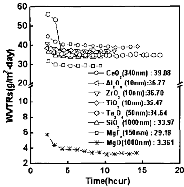
그림 2. PC 필름에 증착된 무기 박막의 투습율 그래프.
