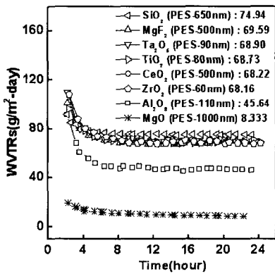
그림 3. PES 필름에 증착된 무기 박막의 투습율 그래프.
