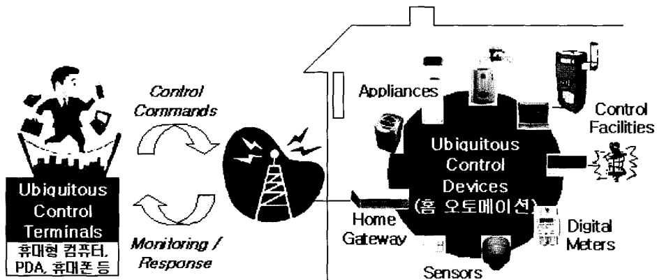
[그림 1] 스마트 홈 유비쿼터스 컨트롤 시스템의 구성
