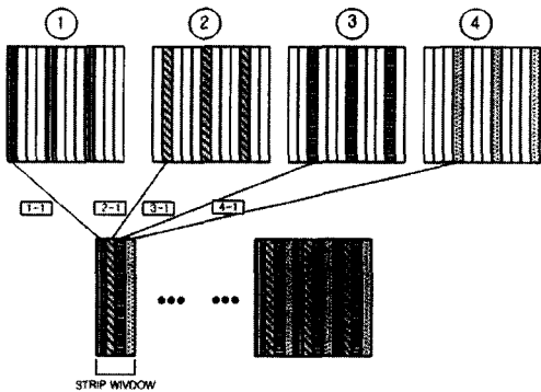
그림 4. 4시점 영상으로부터 스트립 패턴영상의 합성과정
