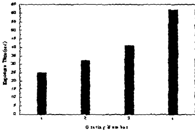
그림 10. 회절화된 4개 격자의 노출시간
