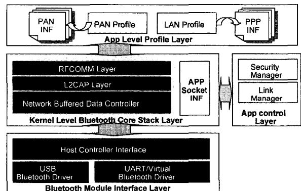
(그림 5) 블루투스 프로토콜 스택 구조도
