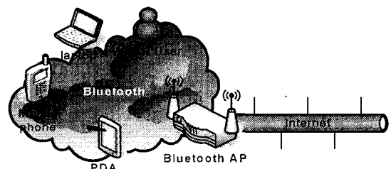
(그림 1) 블루투스 액세스 포인트 구성도
