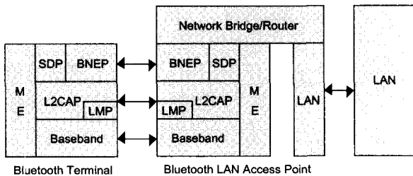
(그림 9) 블루투스 PAN 구조도
