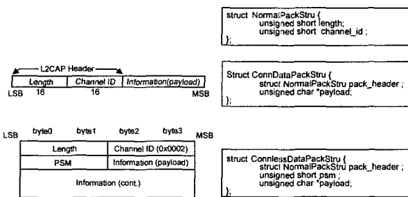
(그림 6) L2CAP 계층 데이터 패킷 구조체
