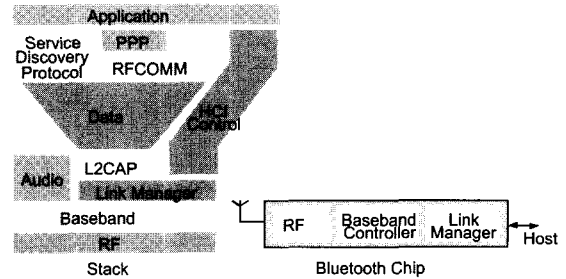
(그림 2) 블루투스 스택과 칩 구조도
