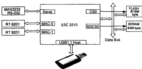
(그림 4) 하드웨어 시스템 블록도
