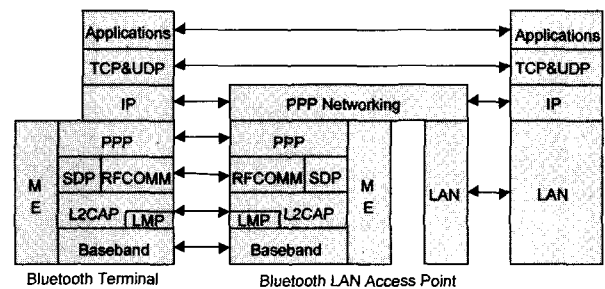
(그림 7) 블루투스 LAP 구조도
