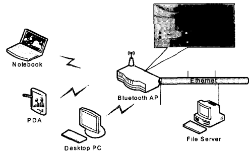
(그림 11) 시스템 실험 환경도
