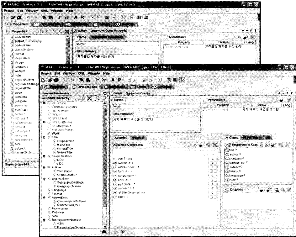
〈그림 5〉 Protege 2.1을 이용하여 생성한 서지 온톨로지
