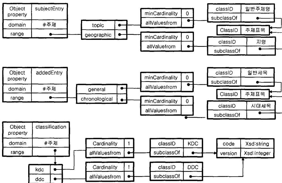
<그림 4> '주제' 클래스 관련 OWL 모델링
