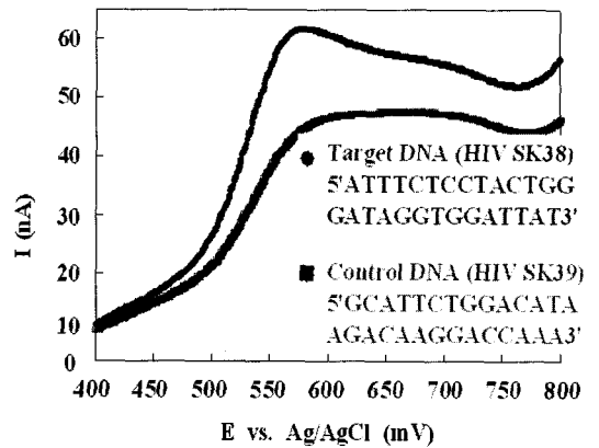
그림 10. Target DNA와 mismatched DNA의 hybridization후 Hoechst 33258의 LSV.
