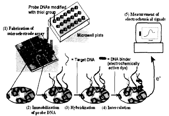
그림 3. 전기화학계를 이용한 DNA칩의 원리. Fig. 3. Principle of DNA chip using electrochemical system.
