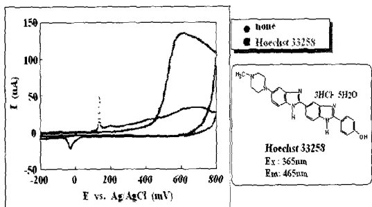
그림 5. 마이크로전극어레이에서 Hoechst 33258의 CV.
