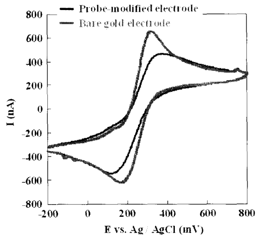
그림 8. Probe DNA 수식된 전극의 CV.
