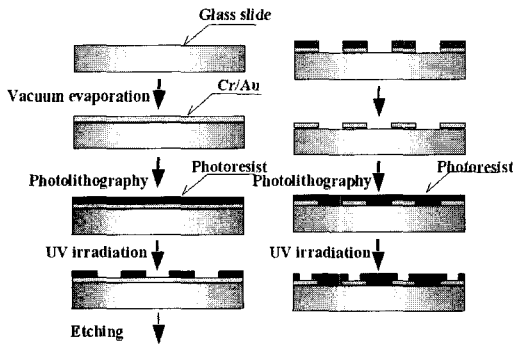
그림 1. 마이크로전극어레이의 제작 공정. Fig. 1. Fabrication process of microelectrode array.
